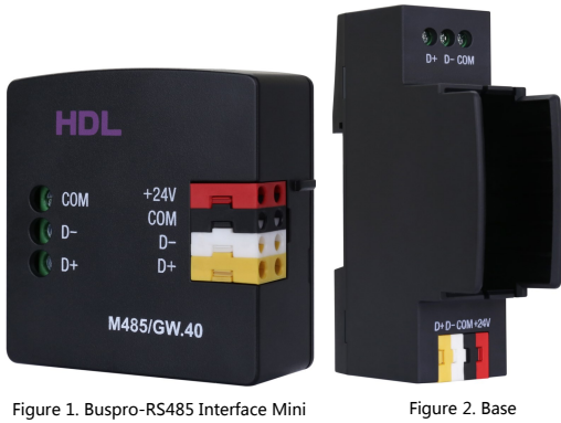
Figure 1. Buspro-RS485 Interface Mini
