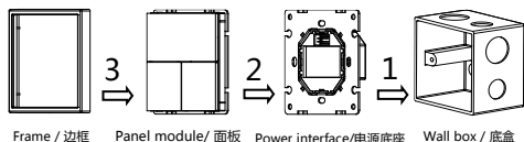
Figure 6. Installation 图 6. 安装图
